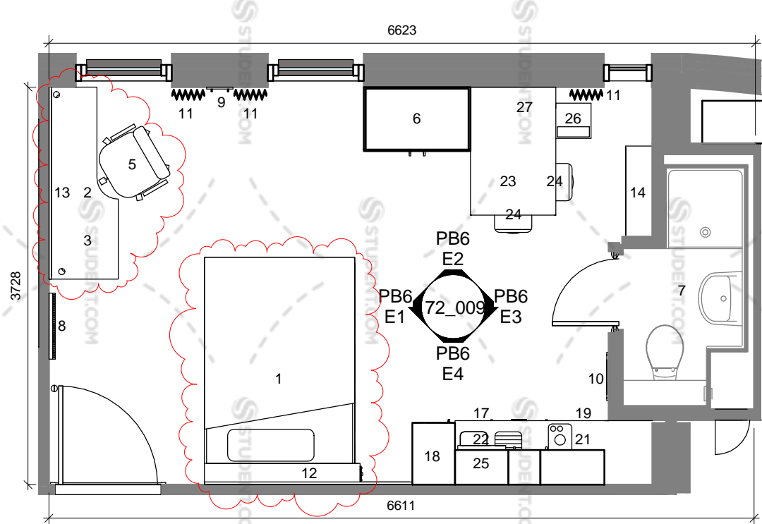
Premium Bedroom 6 Plan 1 : 50
